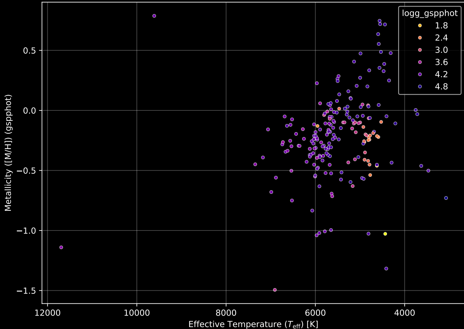
APOGEE DR17 Field: [171-52_MGA] Stellar Population Parameters (n= 200)
